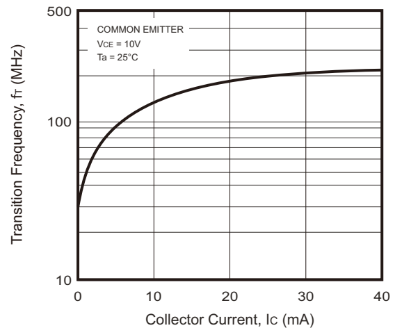
Fig.6 - f_T — I_c
