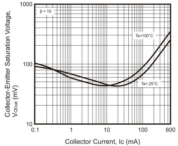
Fig.4 - V_{CEsat} — I_c
