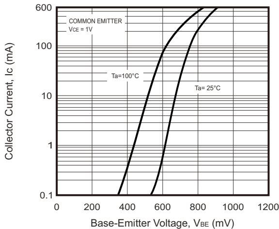
Fig.5 - I_c — V_{BE}
